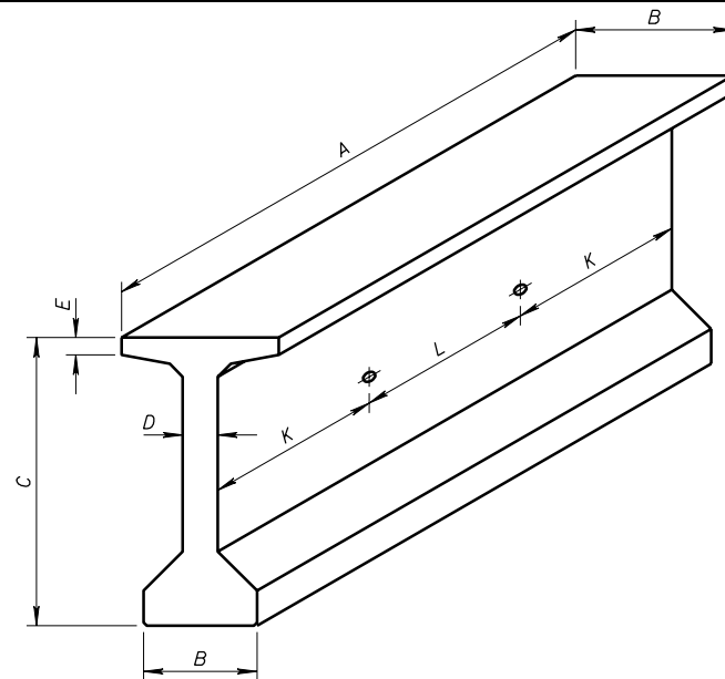
AASHTO MODIFIED TYPE 4 BEAMS
