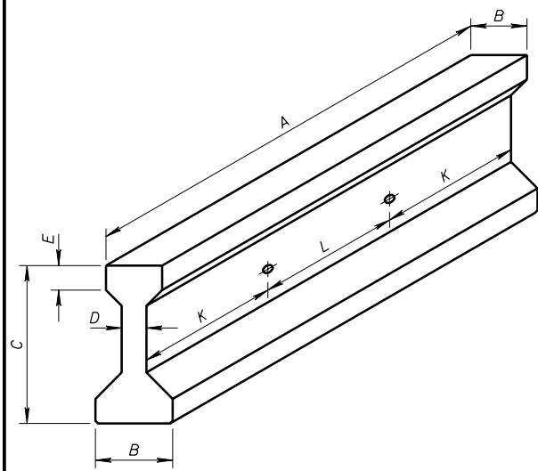
AASHTO TYPES 2, 3 & 4
