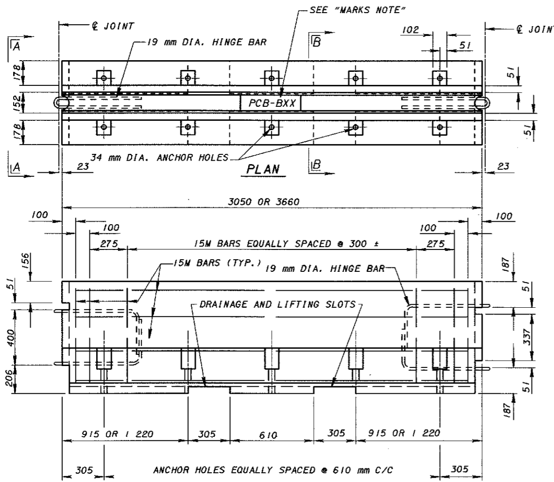
ELEVATION
