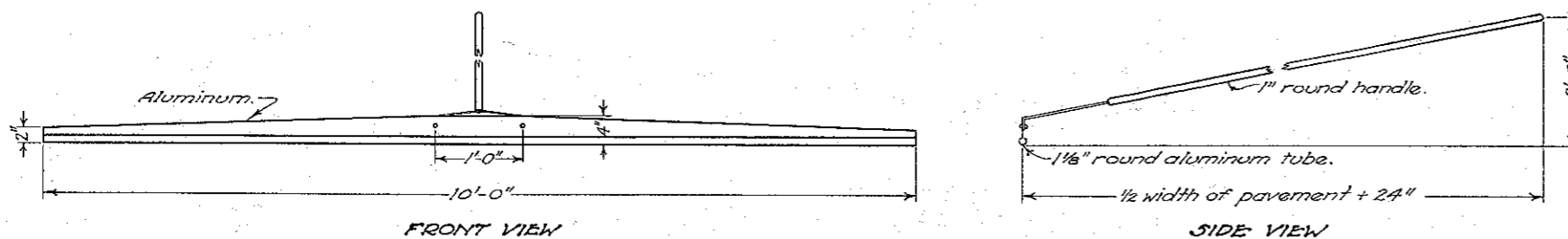
ALUMINUM STRAIGHT EDGE
